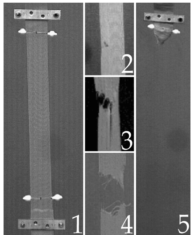
Figura 2 Fotogramas de diferentes instantes de los ensayos mecánicos de tracción aplicados sobre el vendaje neuromuscular obtenidos mediante una cámara de vídeo de alta velocidad Motion Scope™ M1 (Red Lake, EE. UU.). En el fotograma 1 se aprecian las pinzas superior e inferior así como los puntos de digitalización del espécimen. En los fotogramas 2, 3 y 4 se ven diferentes fases de la rotura de la venda una vez superado el punto de máximo esfuerzo. Finalmente, en el fotograma 4 se observa el instante de retracción de la parte superior una vez rota la venda.
