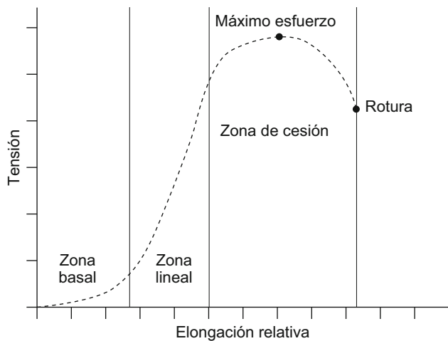
Figura 1 Gráfica típica de tensión/elongación relativa de cualquier material viscoelástico con las zonas típicas: basal, lineal y de cesión. A diferencia del modelo de gráfica que muestran los materiales elásticos (muelle ideal), tan sólo la zona lineal conserva la relación de proporcionalidad entre tensión y deformación.
